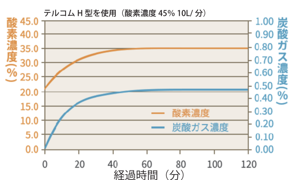
ケージ内ガス濃度変化 (ケージ内容積 250L 体重 5Kg のシュミレーション値)
